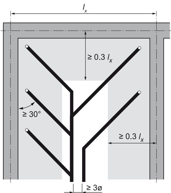
Figura 47 Condotte nelle solette
