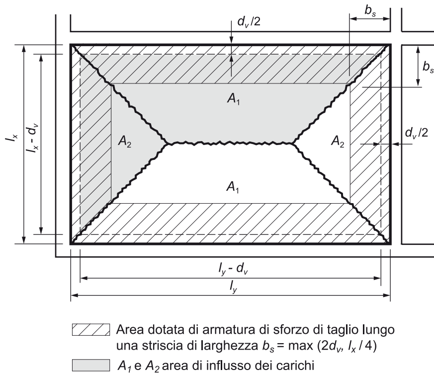
Figura 37 Definizione della sollecitazione della forza di taglio a una distanza di d_v/2 dal bordo dell'appoggio e nelle aree con armatura di taglio
