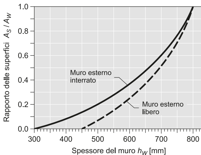
Figura 10: Spessore della parete esterna
