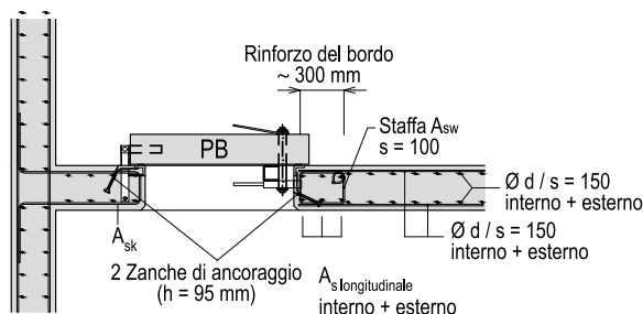
Figura 56: Dettaglio della porta blindata
