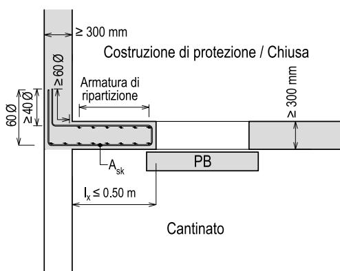
Figura 55: Mensola a parete
