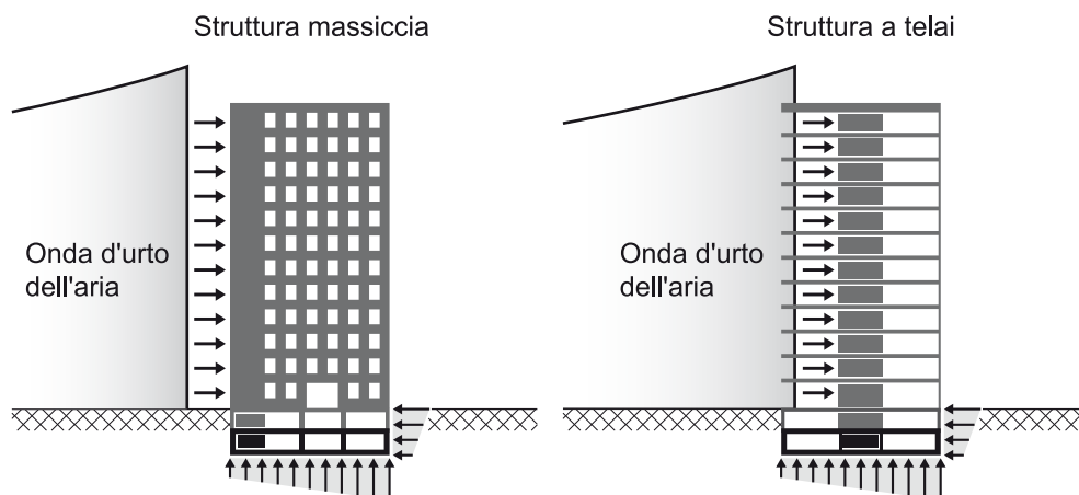
Figura 1 Azione dell'onda d'urto sugli edifici
