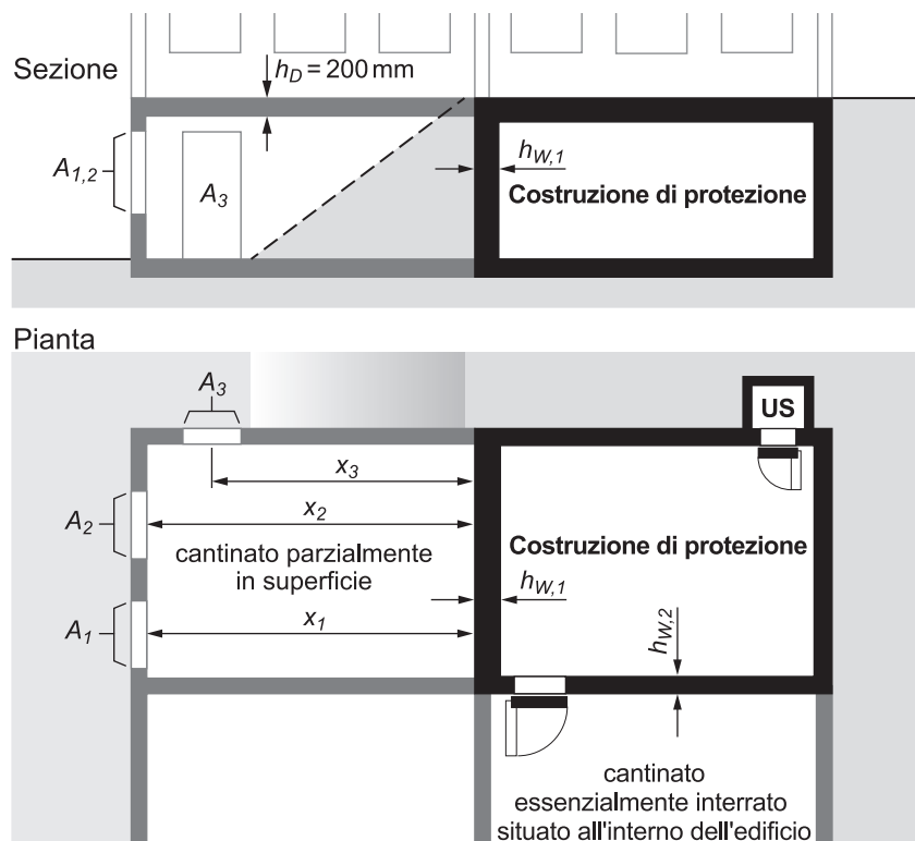
Figura 12: Esempio di dimensionamento degli spessori delle pareti per una costruzione di protezione con cantinato
