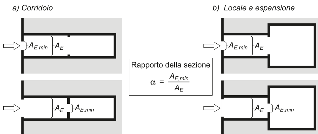
Figura 26 Definizione del rapporto di sezioni \alpha
