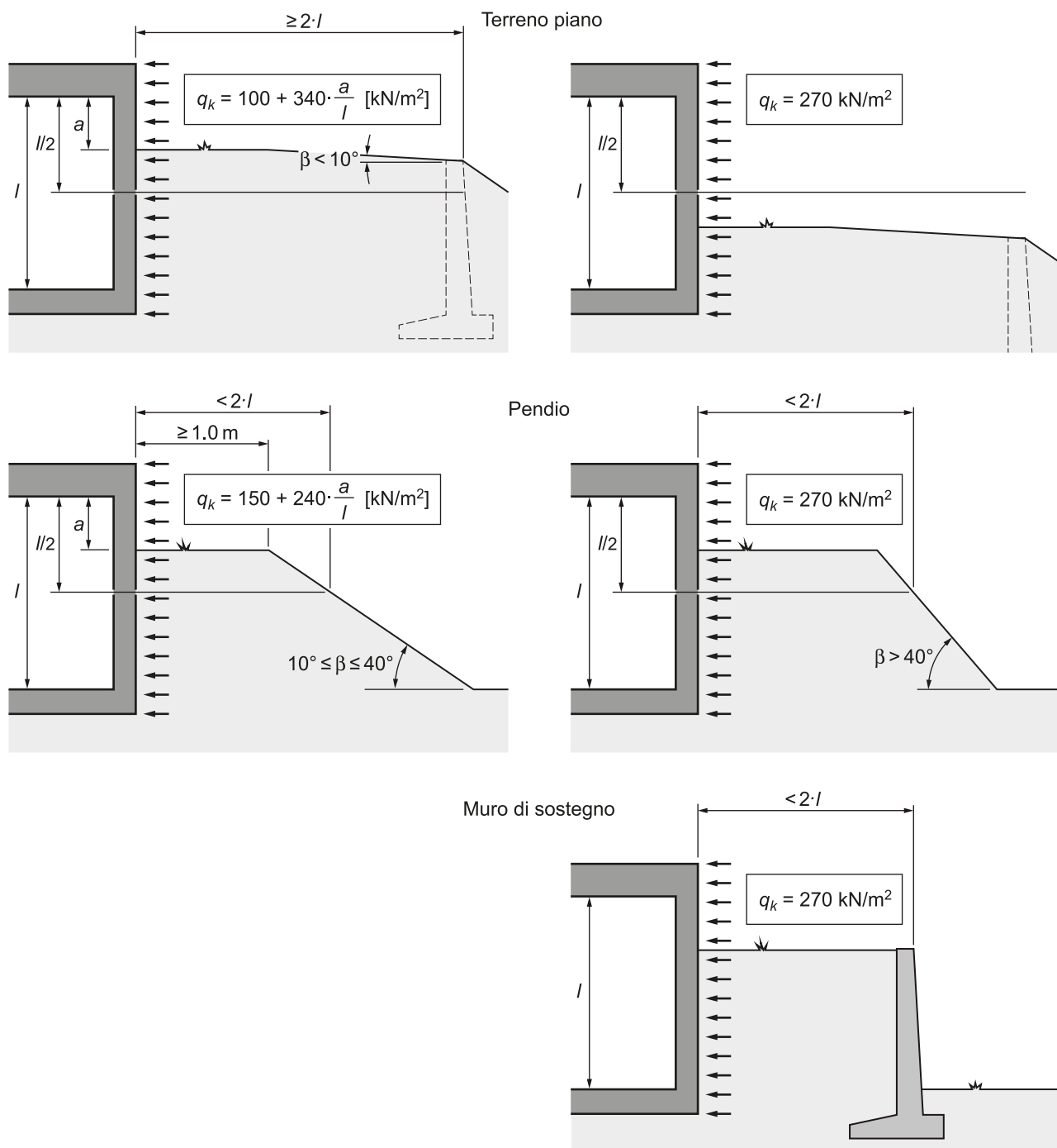
Figura 22 Azione dovuta all'onda d'urto e all'onda sismica indotta nel terreno sulle pareti perimetrali interrate per superfici prevalentemente piane e di scarpate e di muri di sostegno.
