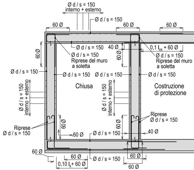
Figura 61 Sezione della chiusa con un'armatura della soletta alternativa a quella illustrata alla Figura 59 (staffe nelle pareti non indicate)
