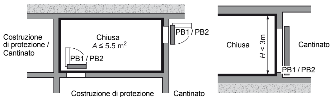
Figura 53: Elementi strutturali di una chiusa
