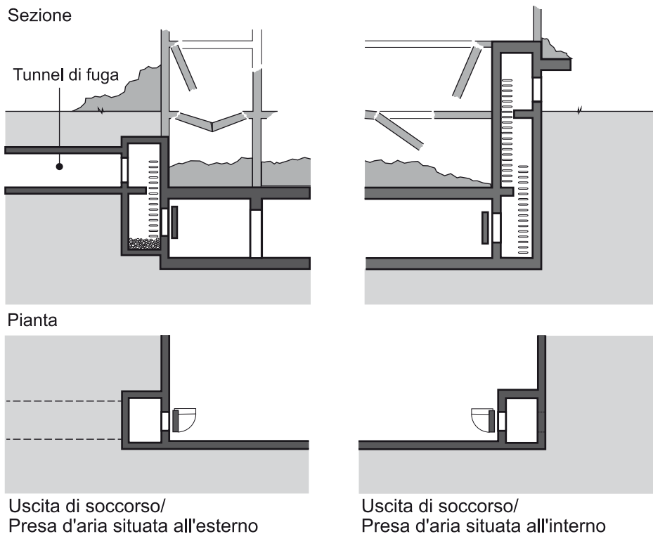
Figura 32 Uscite di soccorso e prese d'aria delle costruzioni di protezione situate sotto vari piani interrati non protetti
