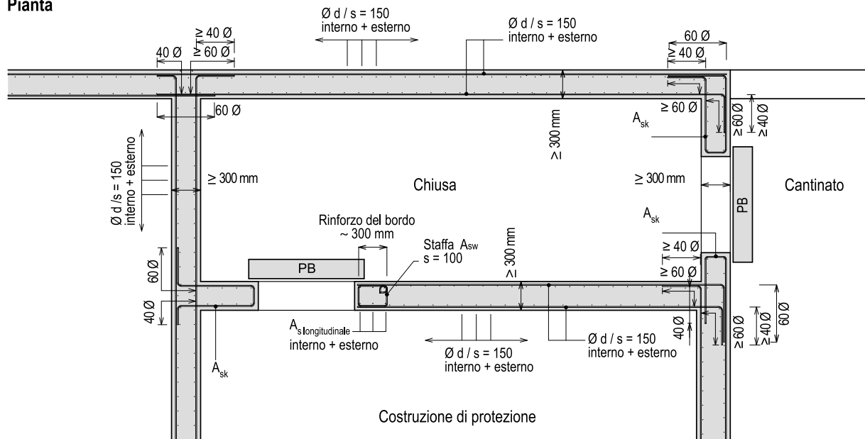
Figura 58 Pianta dell'armatura parete (staffe nelle pareti non indicate)
